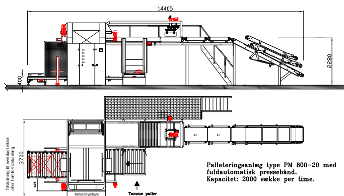
Layout C. Målestok 1 : 200
